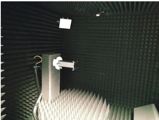
コンパクトアンテナテストレンジ内部
