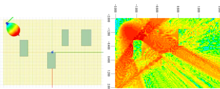
28GHzの電磁波の伝搬の解析結果
